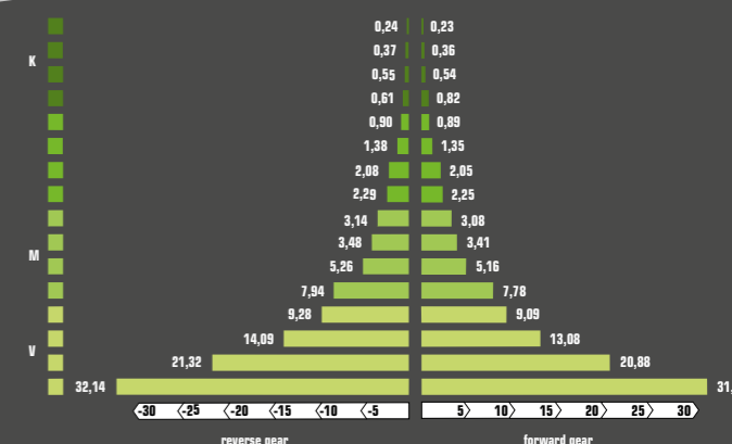
Jemné dávkování: snadné ovládání otáček motoru spojené s dostatkem převodů patří mezi další z vlastností, které dělají z Agrokidu plnohodnotný traktor.
